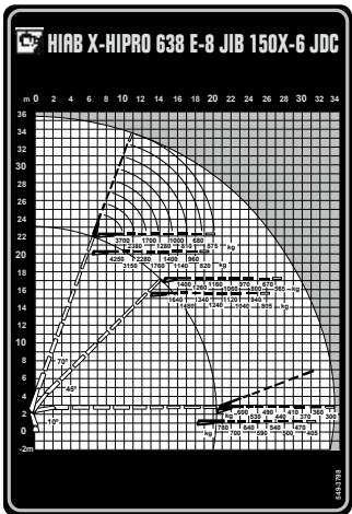
Diagrama de carga HIAB X-HIPRO 638 E-8 JIB150X-6
