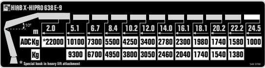
Placa de capacidade HIAB X-HIPRO 638 E-9
