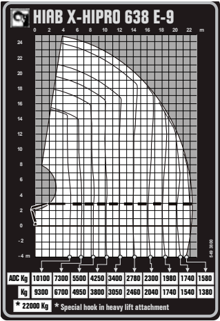
Diagrama de carga HIAB X-HIPRO 638 E-9
