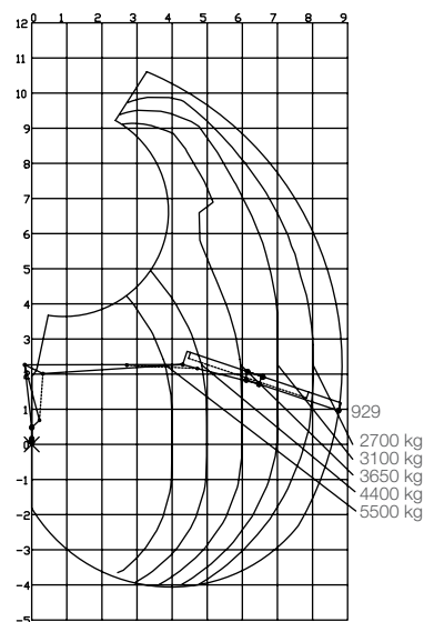
Kuormitustaulukko F251S88C
