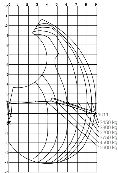
Kuormitustaulukko F251S89A
