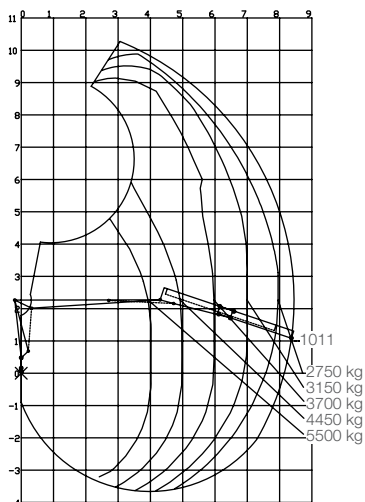
Kuormitustaulukko F251S84C
