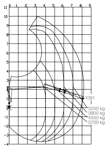
Kuormitustaulukko F251S82A
