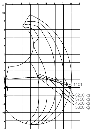
Kuormitustaulukko F251S79C
