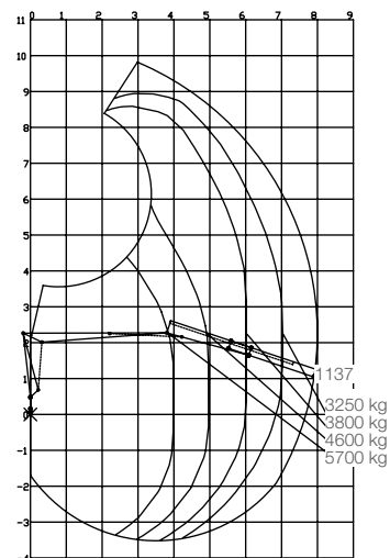
Kuormitustaulukko F251S80A
