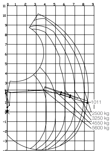
Kuormitustaulukko F251S84A
