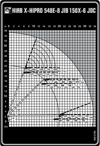
Diagrama de carga HIAB X-HIPRO 548 E-8 + JIB 150X-6 JDC
