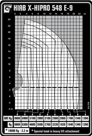
Diagrama de carga HIAB X-HIPRO 548 E-9
