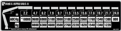
Placa de capacidade HIAB X-HIPRO 548 E-9
