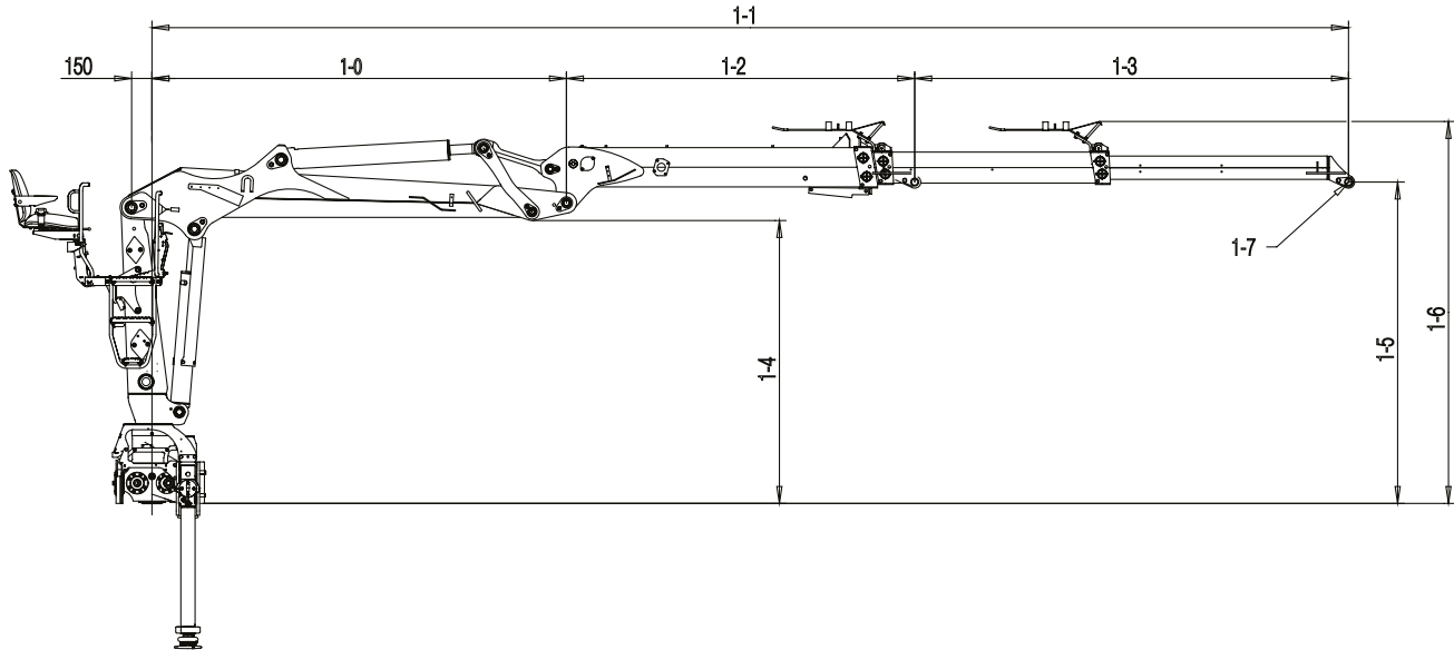
Vista lateral
