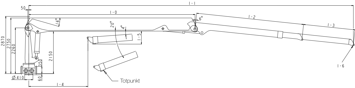
Seitenansicht
