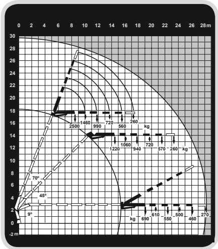
Diagramme de charge HIAB X-HIPRO 352 E-6 JIB 70X-4
