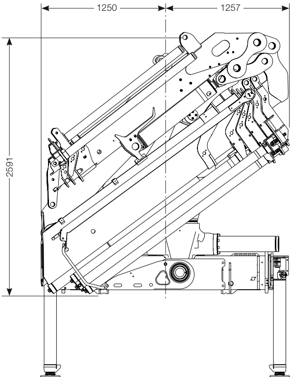
Schéma de vue latérale HIAB X-HIPRO 352
