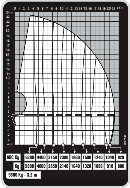
Diagramme de charge HIAB X-HIPRO 352 E-8
