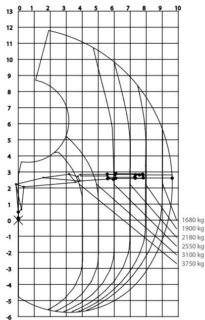
Lastdiagramm F140S 96 BOOSTER
