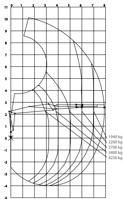
Lastdiagramm F140S 79
