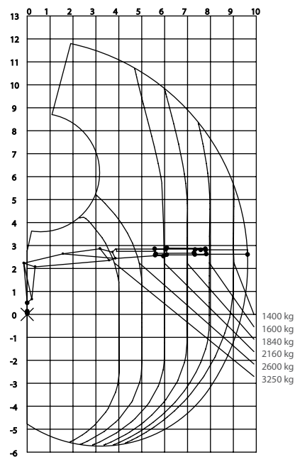
Lastdiagramm F140S 96
