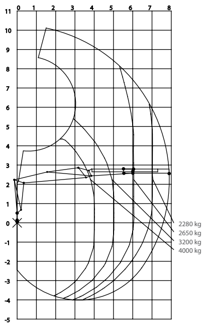
Lastdiagramm F140S 79 BOOSTER
